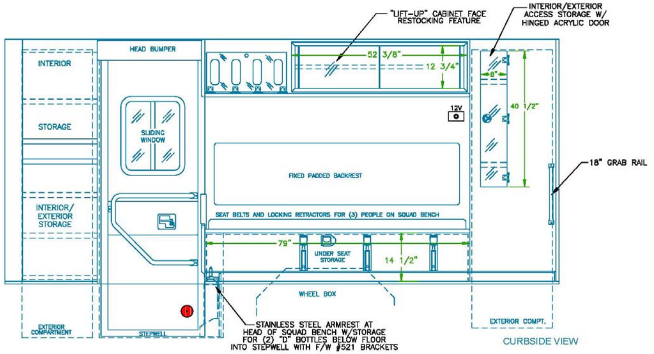
Curbside Layout
